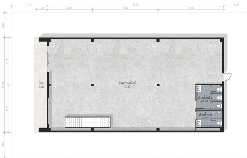
รายละเอียดอาคารพาณิชย์ ควบคุมอาคาร พ.ศ.2543 1st FLOOR PLAN
